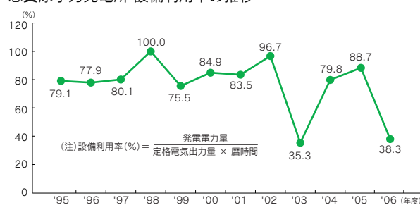
志賀原子力発電所 設備利用率の推移
