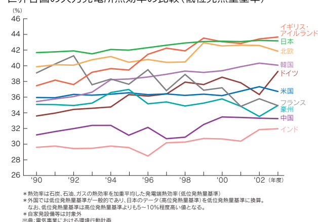
世界各国の火力発電所熱効率の比較(低位発熱量基準)
