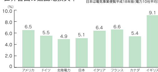
世界各国の送配電損失率
