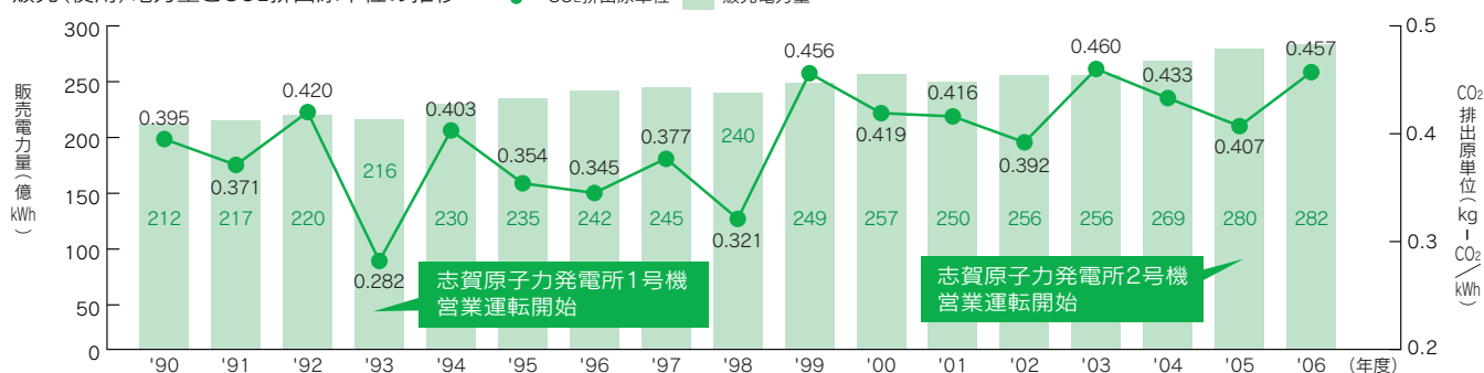
販売(使用)電力量とCO 2 排出原単位の推移
